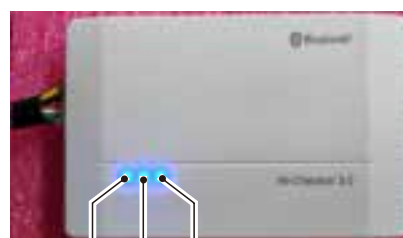
LED3 LED1 LED2
